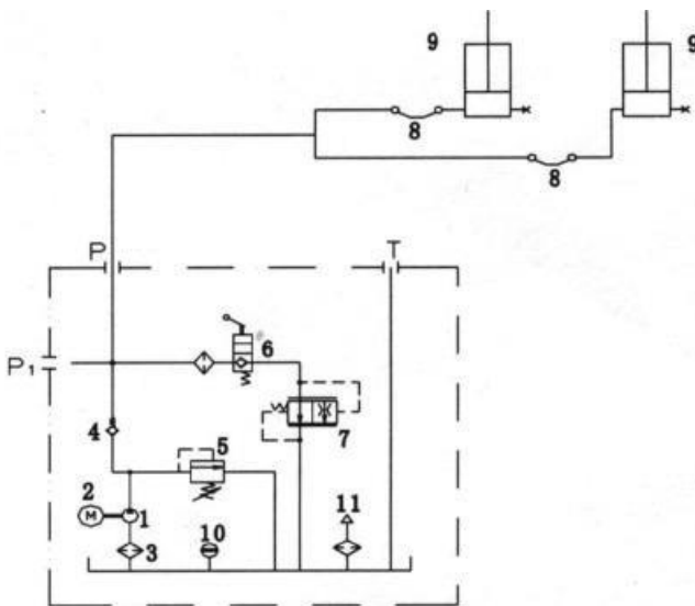
Схема гидролиний
