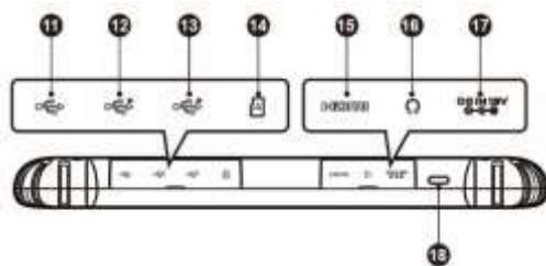
Рисунок 2-3. Диагностический сканер MaxiSys (вид сверху)
