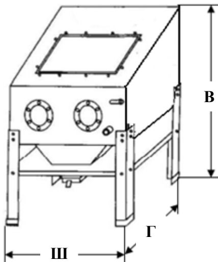
Рис. 1. Габаритные размеры установки
