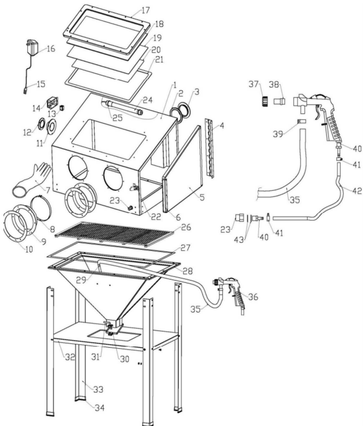
Рис. 3. Устройство изделия.
